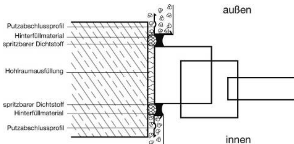
Bild 6: Fachgerechte Fugenausbildung nach erfolgtem Putzauftrag.
