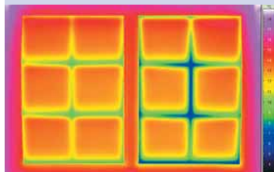
▲ Infrarotaufnahme: Kunststofffenster mit Sprossen links: mit sgg SWISSPACER-Abstandhalter und Wiener Sprosse rechts: normaler Alu-Abstandhalter mit Aluminium-Sprossen
